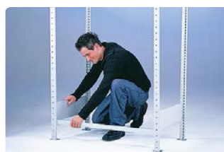
... durch Kreuzstrebe (6) mit Spannschloss
